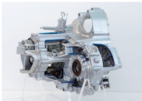
材料から一貫生産している主力製品のトランスミッション
